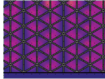
Radiation map με ανοιχτά σκίαστρα-καλοκαίρι
