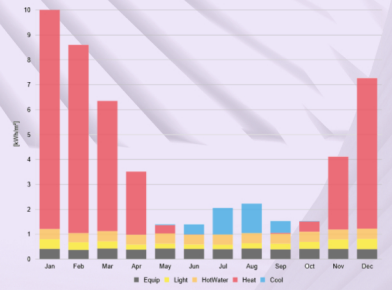
ΜΕΤΡΗΣΗ ΧΩΡΙΣ ΤΟ ΣΥΣΤΗΜΑ ΣΚΙΑΣΗΣ
