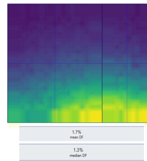
Daylight factor με σκίαστρα
