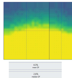
Daylight factor χωρίς σκίαστρα
