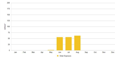
Radiation map- χωρίς σκίαστρα (καλοκαίρι)
