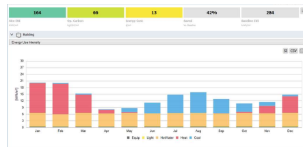
Ενεργειακή κατανάλωση με κλειστά σκίαστρα
