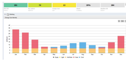
Ενεργειακή κατανάλωση με ανοιχτά σκίαστρα
