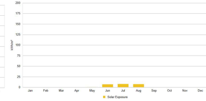
Radiation map- με σκίαστρα (καλοκαίρι)
