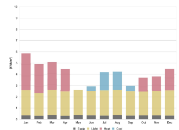
Απαιτήσεις θέρμανσης και ψύξης χώρου
