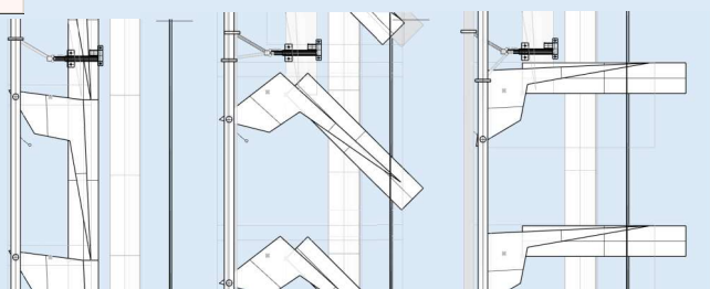
ΤΟΜΗ ΠΟΥ ΔΕΙΧΝΕΙ ΤΗΝ ΚΙΝΗΣΗ ΤΟΥ ΜΗΧΑΝΙΣΜΟΥ (ΙΣΧΥΕΙ ΚΑΙ ΓΙΑ ΤΙΣ ΚΑΘΕΤΕΣ ΚΑΙ ΓΙΑ ΤΙΣ ΟΡΙΖΟΝΤΙΕΣ ΠΕΡΣΙΔΕΣ)
